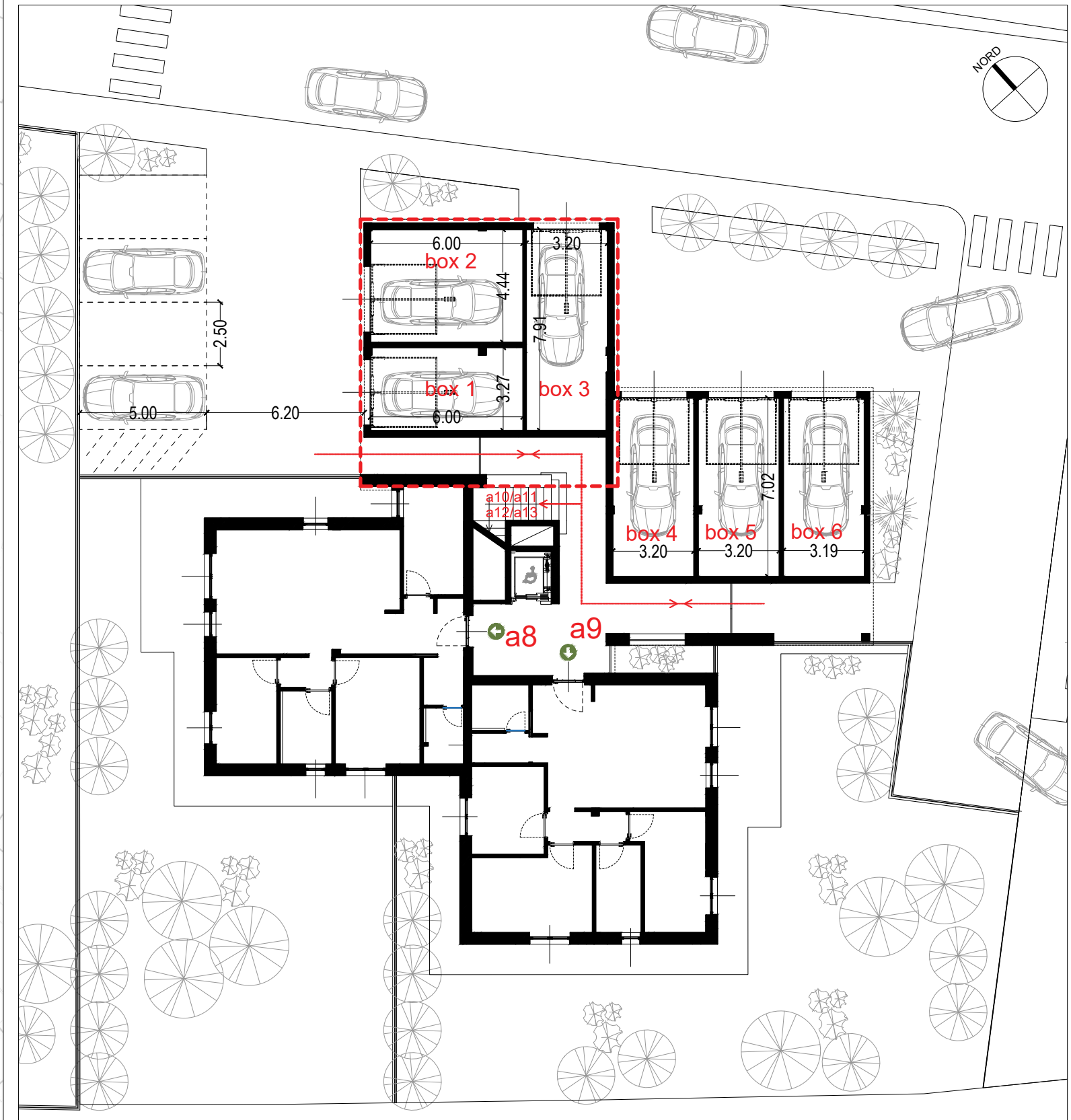
Planimetria (pt)
